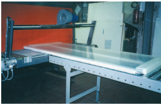
Possibilità di chiusura totale dei lati del pacco, mediante sovrapposizione del film (anche con pacchi di grandi dimensioni).
