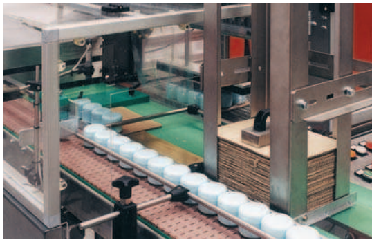
Inserimento automatico di cartoncino piano, per irrigidire i pacchi e migliorare la palettizzazione.
